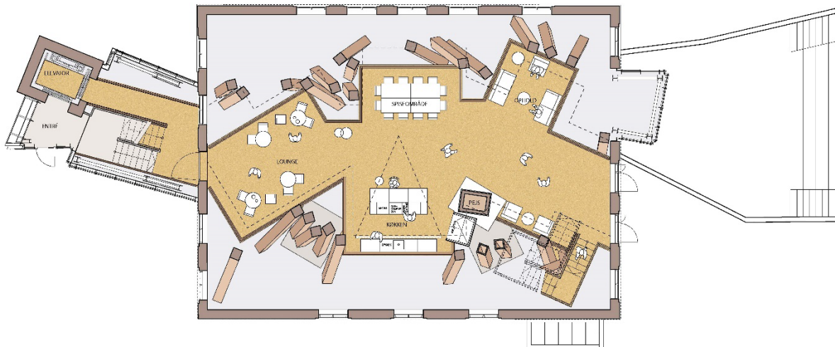
Hejmdal Stueplan, 1:100
