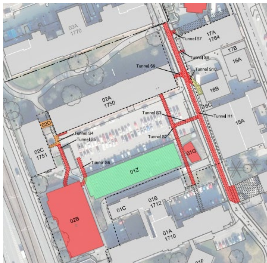
Figur 2: Oversigt over tunneller og bygninger, der skal fjernes.
